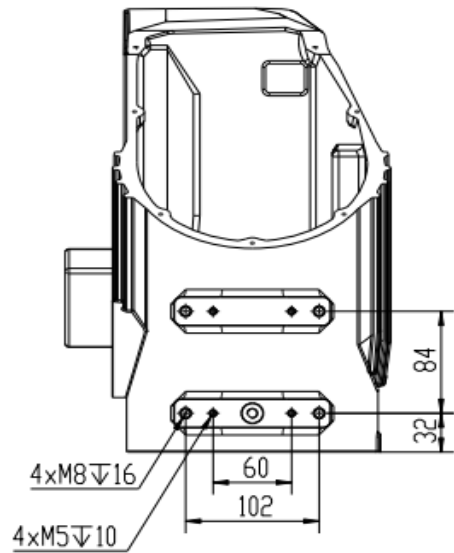
J4电机座安装尺寸 ◀
