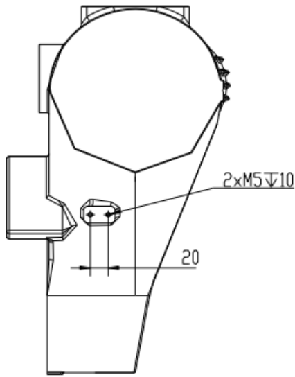
J2转座安装尺寸 ◀
