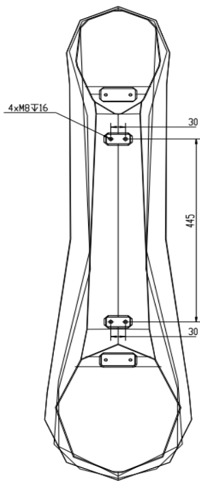
J3大臂安装尺寸 ◀
