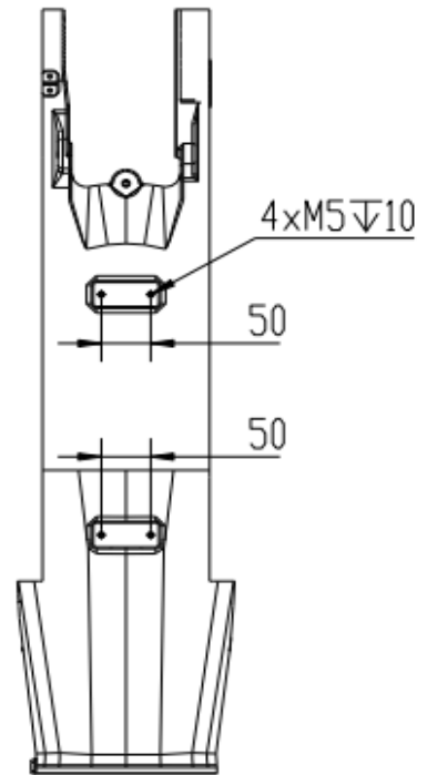
J5手腕体安装尺寸 ◀
